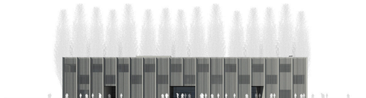
Nordfassade 1:200
