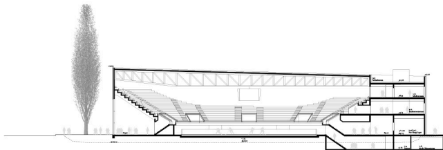
Schnitt AA 1:200
